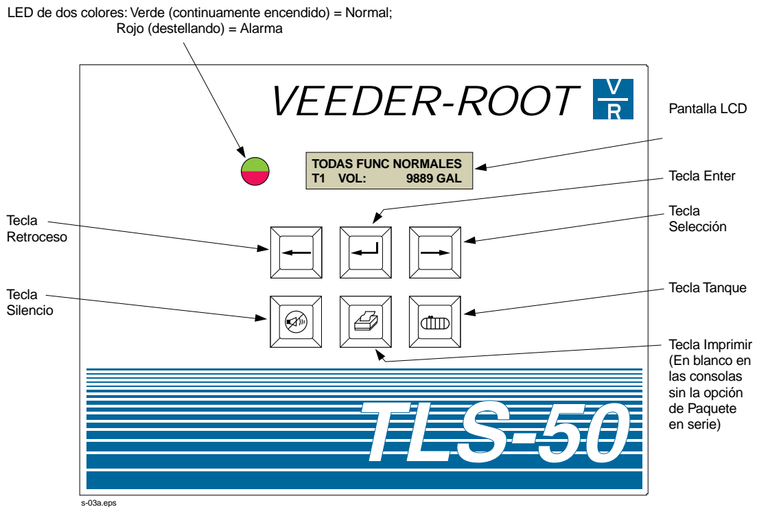
Figura 2. Controles del panel delantero del TLS-50
