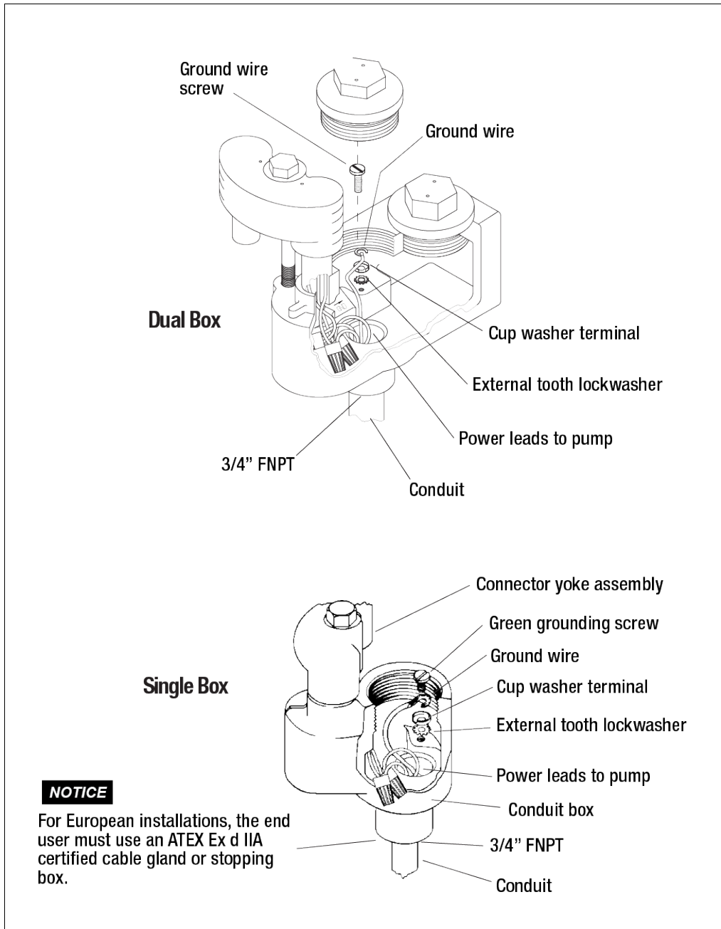
Figure 14. Conduit Box Wiring
